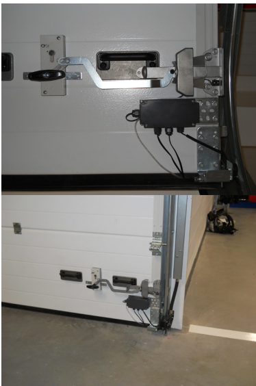
PESTILLO ANTIEFRACCIÓN
